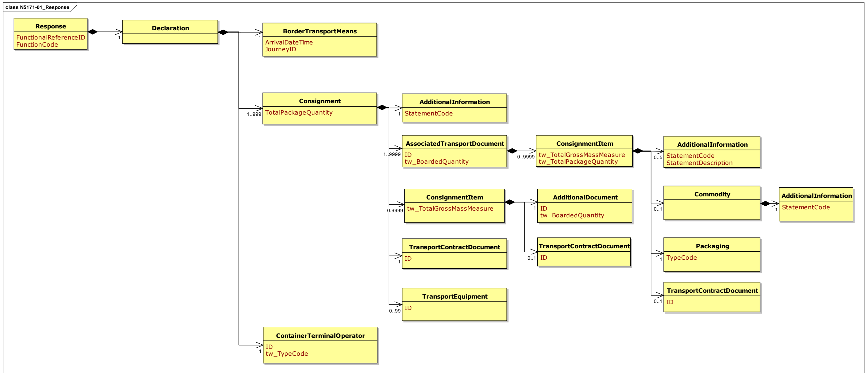
圖 1 訊息類別圖
