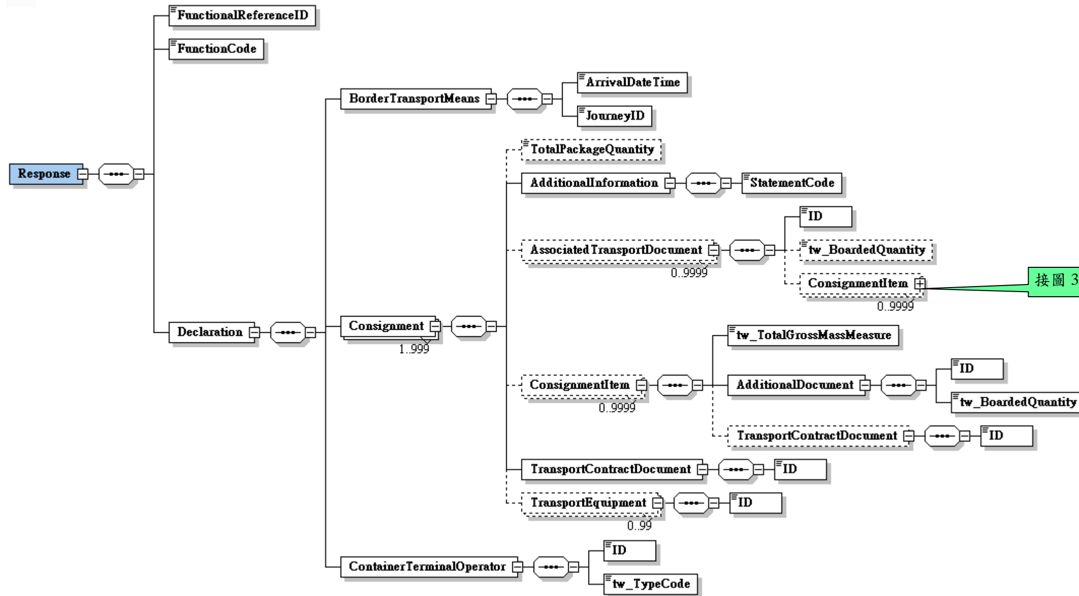
圖 2 訊息架構圖
