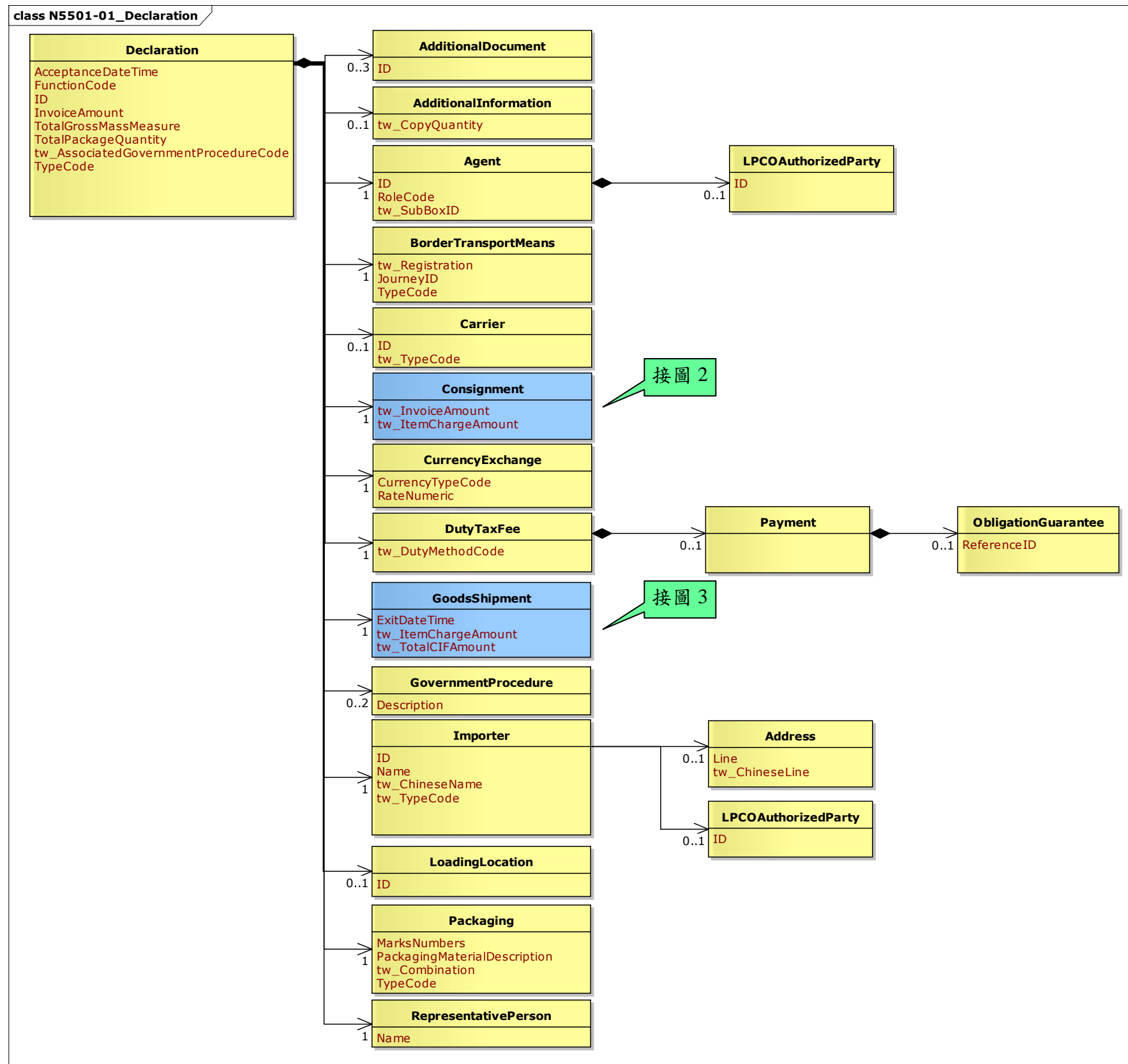
圖 1 訊息類別圖
